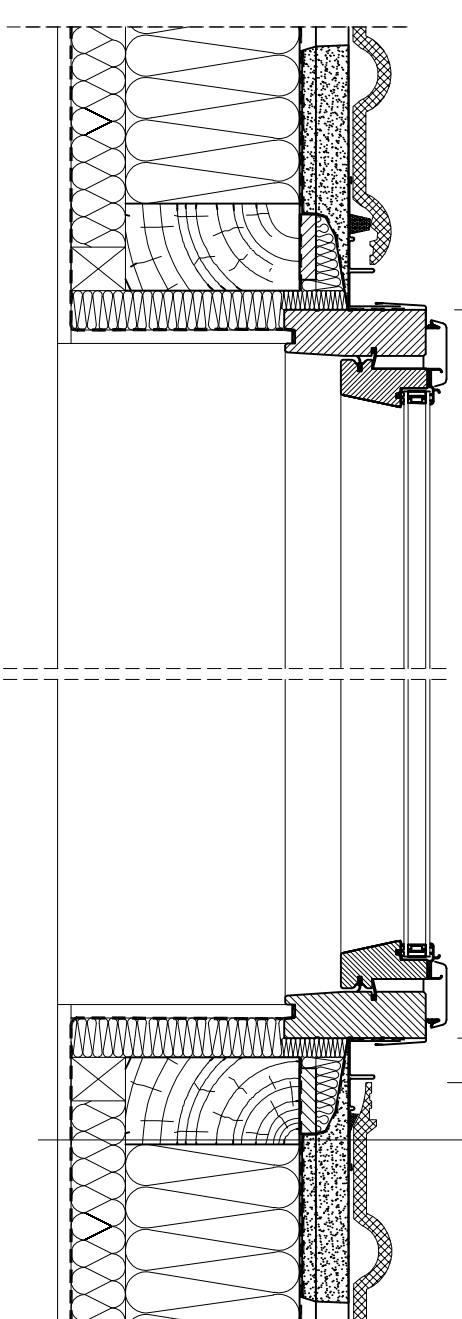
PRZEKRÓJ C - C
